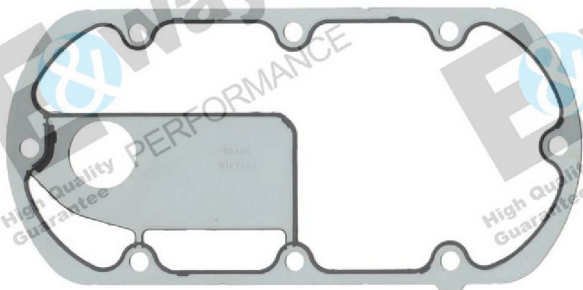
型號: JOHN DEERE/6090/L6/9.0L 原廠號碼: R132396 品名: 冷卻器墊片-外(8孔) 材質: 鐵包橡皮
