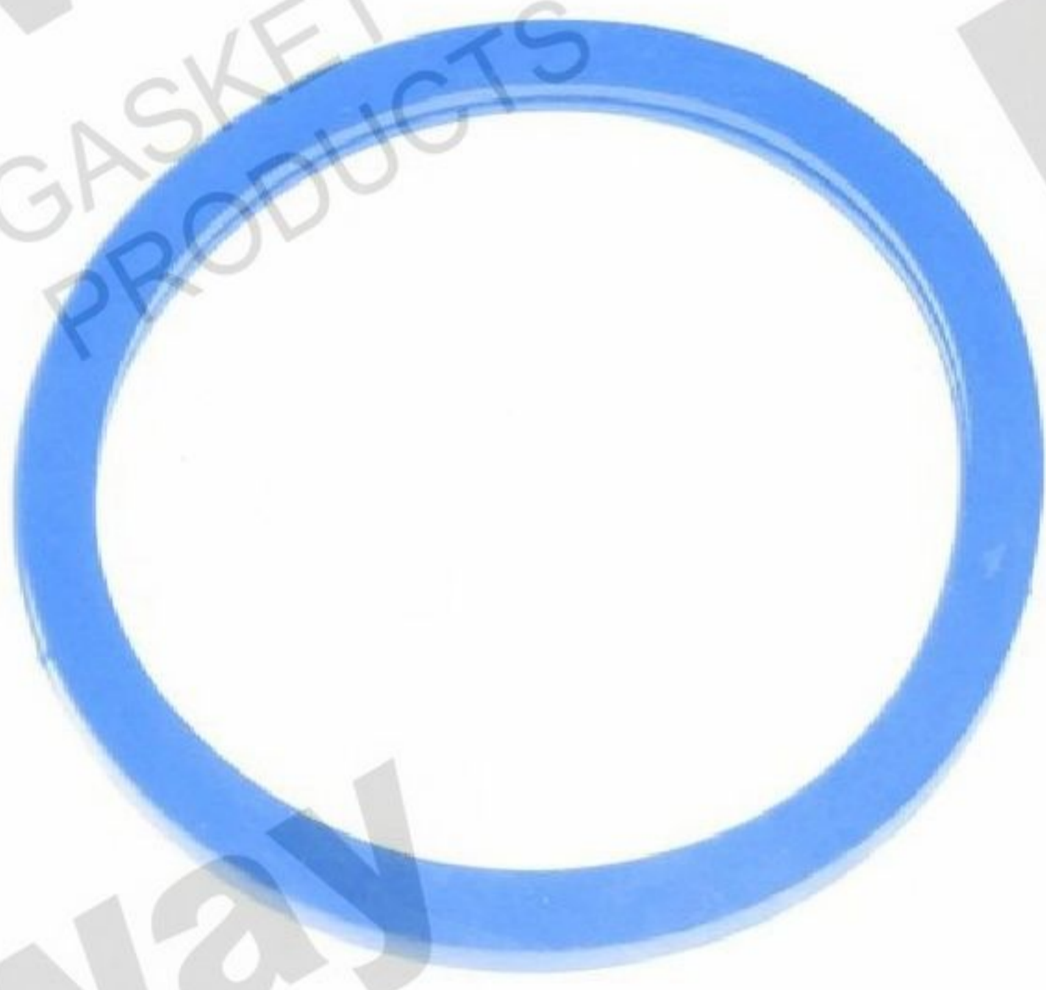
型號: S1632-51400 品名: J08C/J08E水龜座橡皮 材質: NBR
